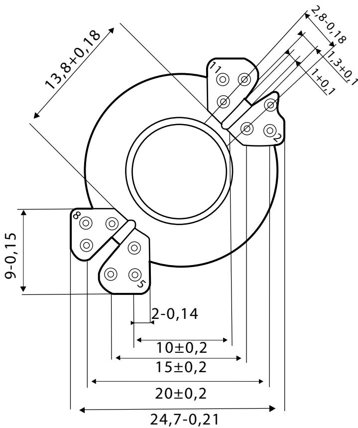
Габаритный чертеж
